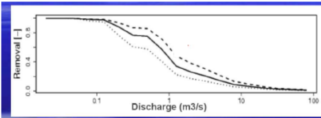
Figure 15 : efficacité d'élimination de l'azote en fonction du débit et de la charge en azote, d'après Wollheim et al. 2008
